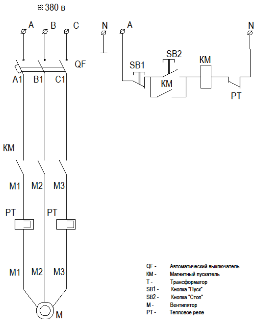
Приложение 1. Схема электрическая принципиальная фильтро-вентиляционной установки ФВУ-01-02.
