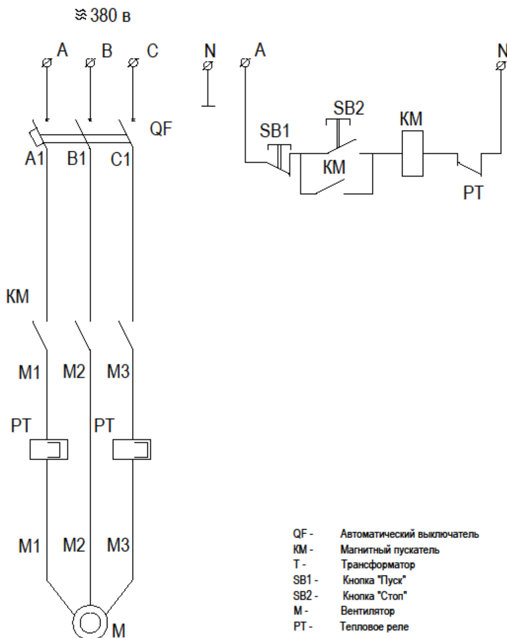
Приложение 1. Схема электрическая принципиальная фильтровентиляционной установки ФВУ-01-04
