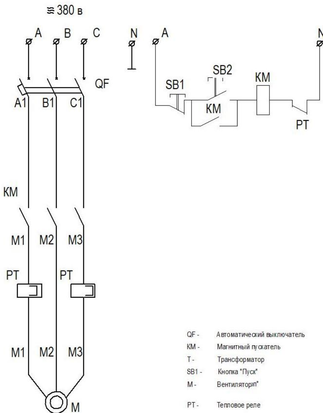
Приложение 1. Схема электрическая принципиальная фильтро-вентиляционной установки ФВУ-03-04
